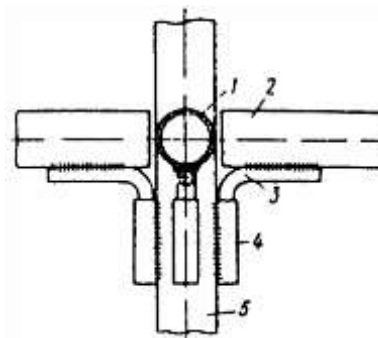
Рис. 2. Узел соединения элементов в безболтовых трубчатых лесах 1 - поперечина; 2 - прогон; 3 - крюк; 4 - патрубок; 5 - стойка
